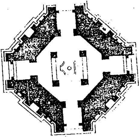
5. मुण्डेश्वरी मंदिर का अष्टमुखी नक्शा (रामगढ़ 7वीं शताब्दी)
