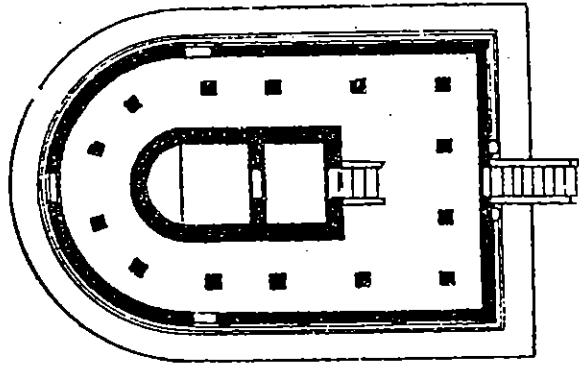
6. वामन मंदिर का अर्द्ध-युतात्मक नक्शा (किष्कावेल्लूर, 11वीं शताब्दी)
