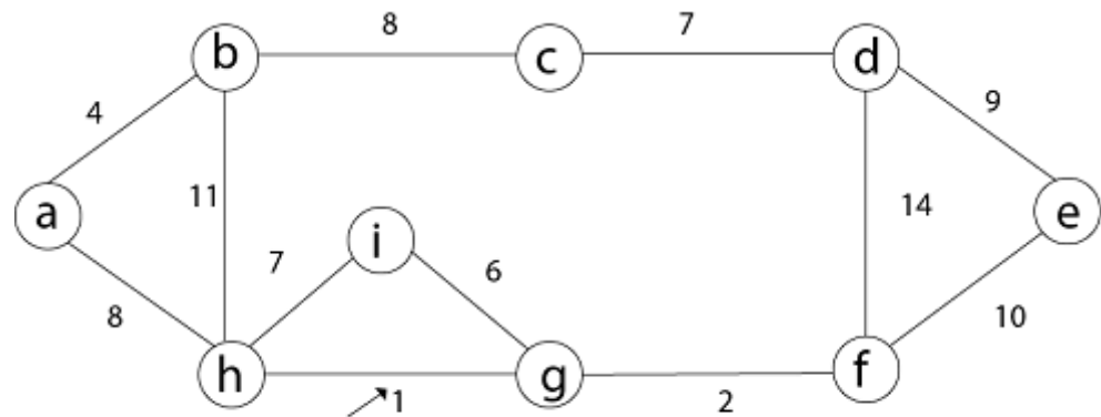
Fig. 4.11 Step-2
