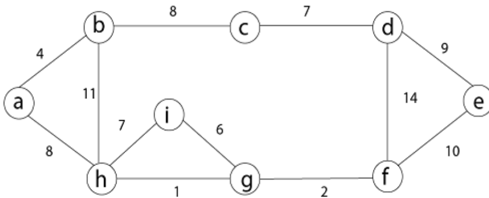
Fig. 4.13 Step-4
