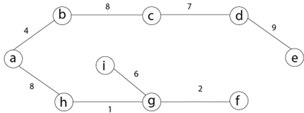
Fig. 4.15 Step-7
