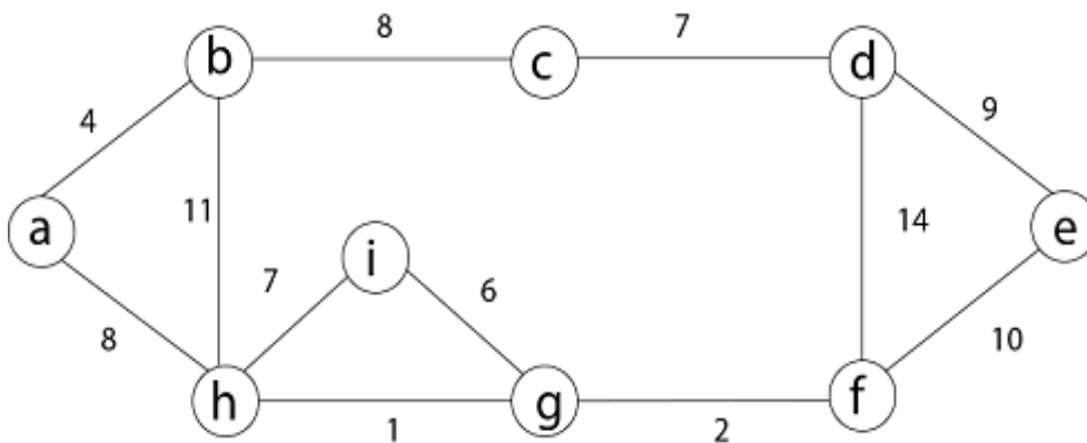
Fig. 4.14 Step-6
