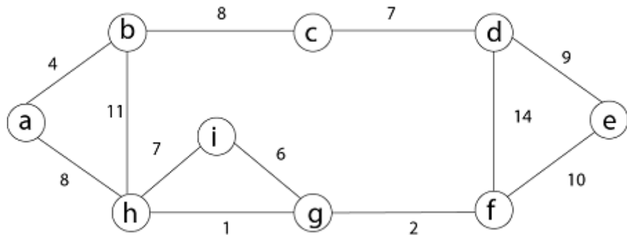
Fig. 4.9 Example
