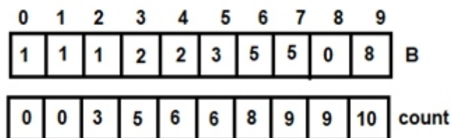
Figure 3.12: For i=8
